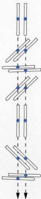
Skienes bevægelse i pivotslips
